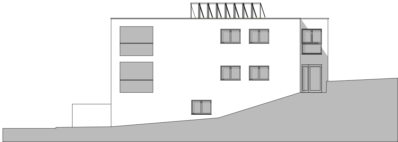
FACCIATA OVEST
