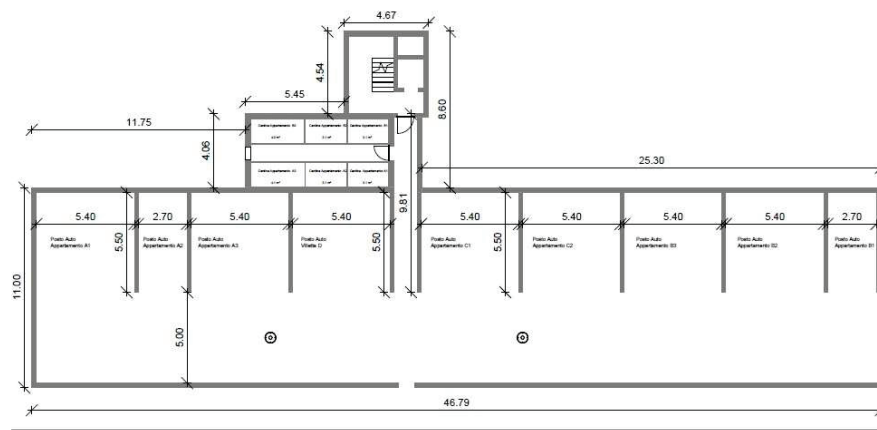
Pianta Autosilo Scala 1:200
