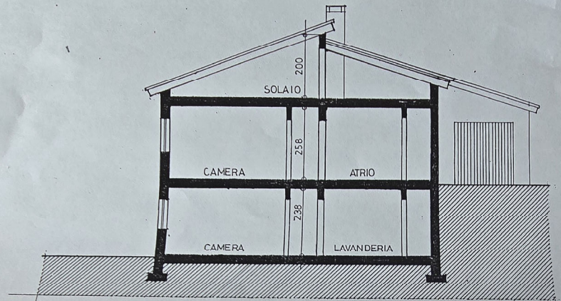
SEZIONE 1
