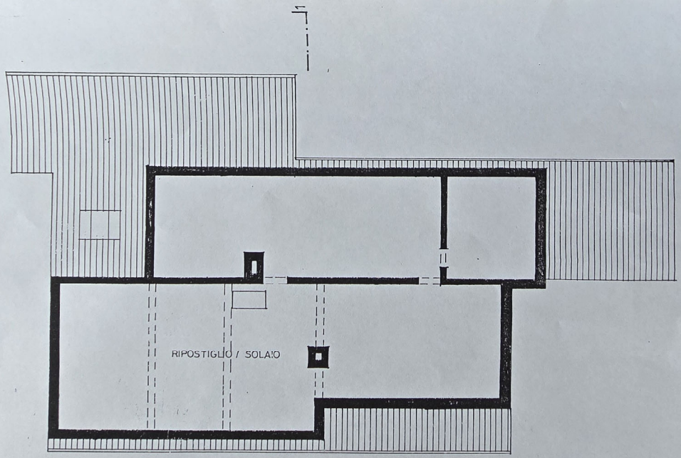
PIANO TETTO
