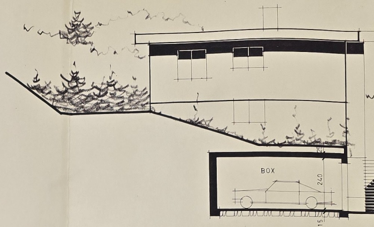
FACCIATA NOR-EST
