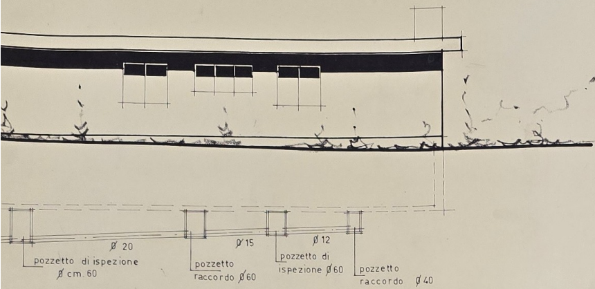
FACCIATA SUD-EST
